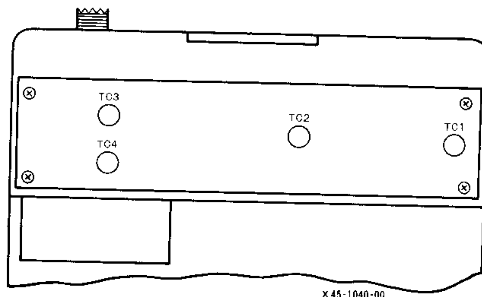
FIG. 10 PA UNIT
